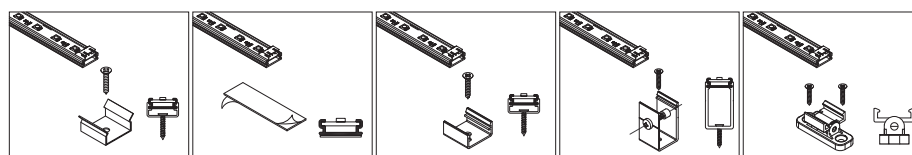
01: Стальной зажим 02: Двусторонний скотч 03: Алюминиевый зажим 04: Алюминиевый зажим (длинный) 05: Угловой зажим
